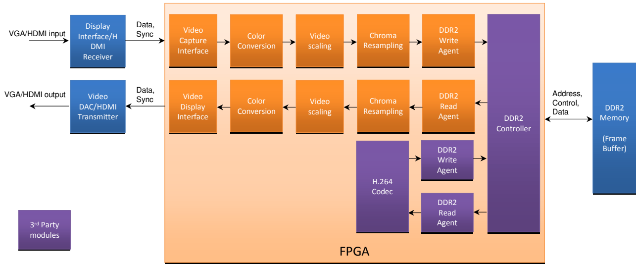
ビデオ処理ユニット ブロック図
